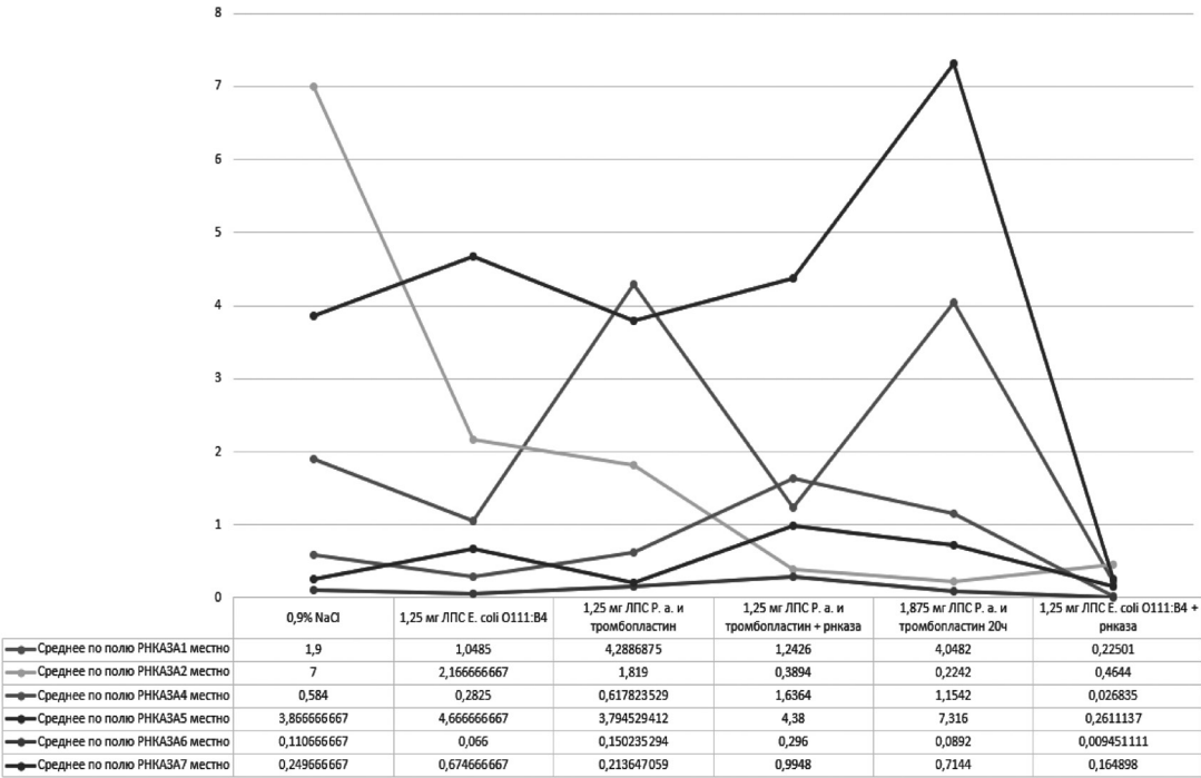
Рисунок 3. Динамика изменения местной экспрессии РНКаза в разных моделях
